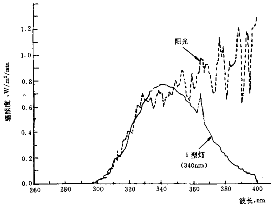
图 A1 峰值 340 nm 的 I 型灯和阳光的比较
